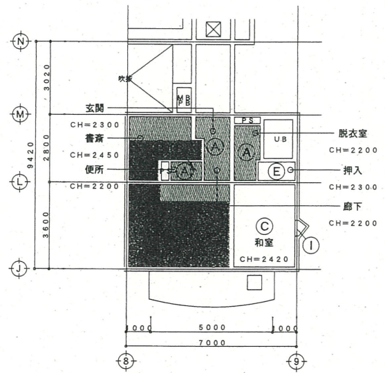
天井伏図 S=1/150
