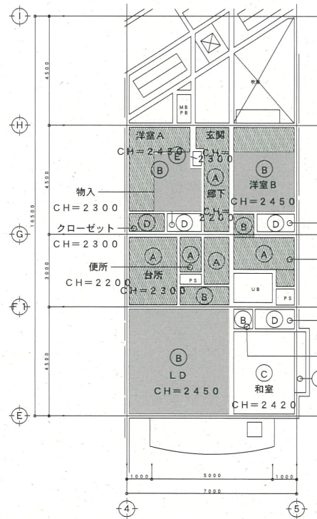
天井伏図 S=1/150
